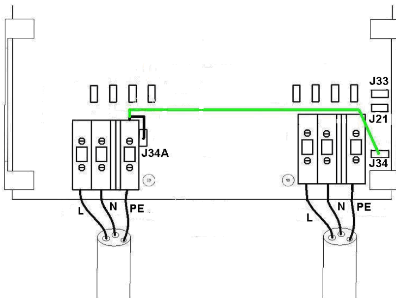
Rys. 4: Podłączenie uziemienia wejścia (w modelu Auto 115/230 V, patrz rys. 4a)
